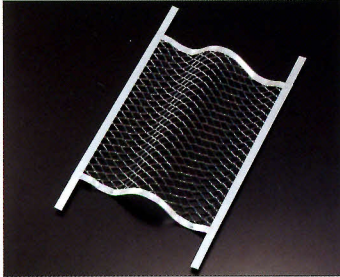
■YKローラーバケットネット (SX・S用 共通)
